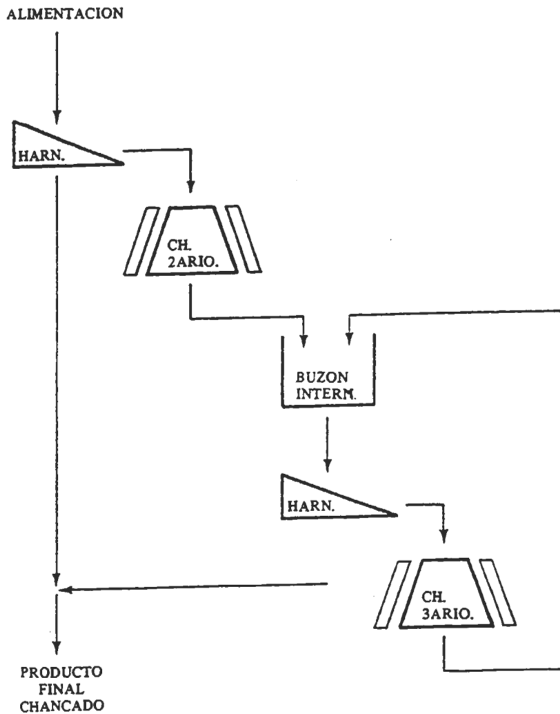
FIGURA 1. CIRCUITO A (ACTUAL DE PLANTA)
