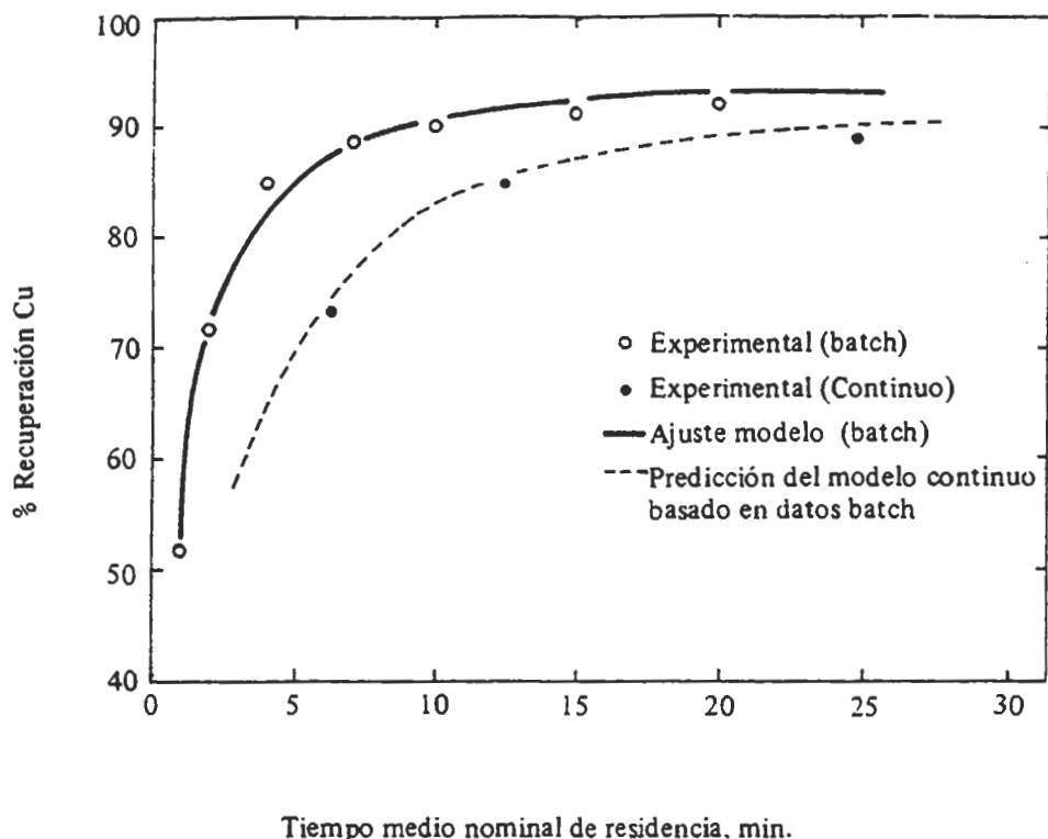
FIGURA 5.9. Simulación de la flotación continua a partir de los datos de laboratorios (Ref. 2.6)
