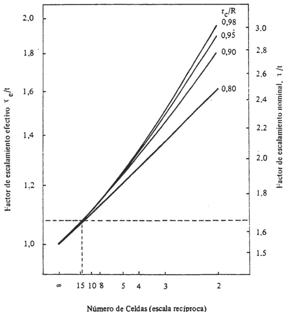
FIGURA 5.8. Factores de escalamiento nominal y efectivo en función del número de celdas. Valores escalados desde laboratorio hasta un banco de celdas Denver No 24. \tau_e = V/Q .
