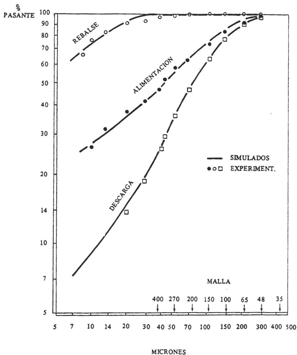
FIGURA Nº 2. RESULTADOS EXPERIMENTALES Y SIMULADOS – TEST Nº 2 Ciclón Krebs - 6" Diámetro Material = Fosfato I ( \rho_s = 2.8 ) Ensayo de Deslamado - Planta Piloto
