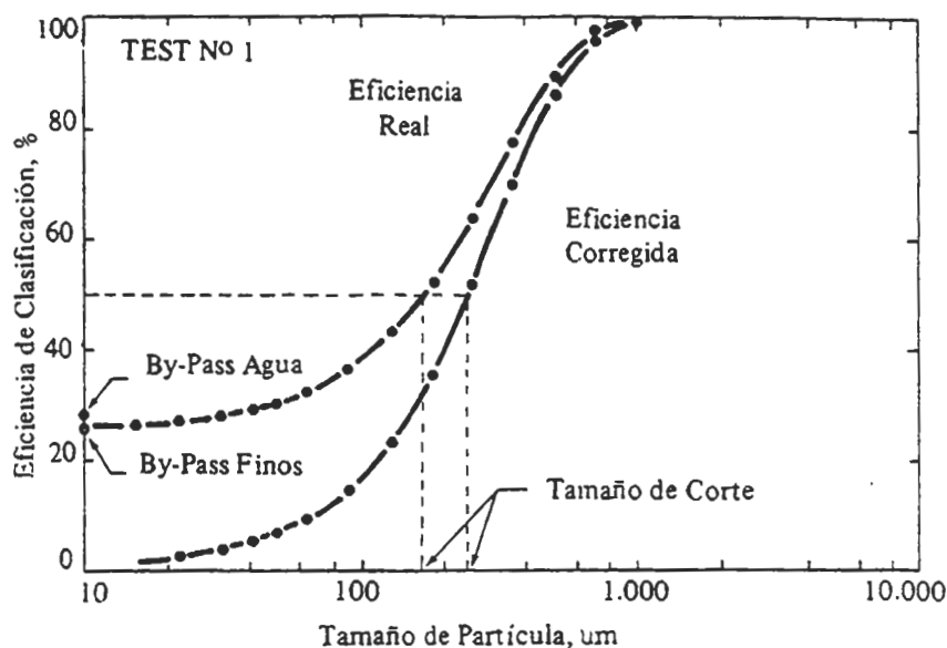
FIGURA 7.— Ejemplo de Curvas de Eficiencia de Clasificación Global y Corregida
