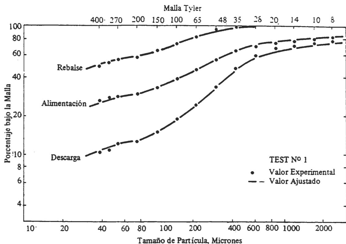
FIGURA 9.— Ejemplo de Curvas Granulométricas ajustadas
