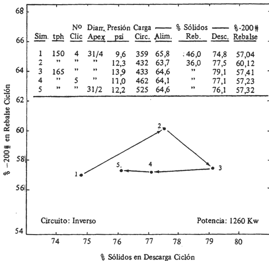
FIGURA 5. Ejemplo de aplicación de técnicas de simulación matemática a la optimización de un circuito tradicional de molienda/clasificación.
