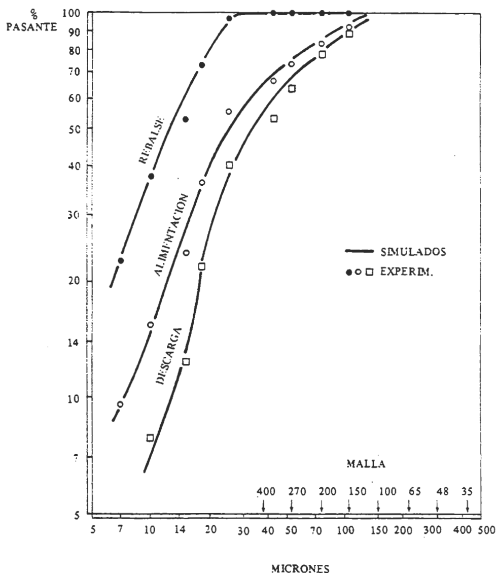
FIGURA Nº 4. RESULTADOS EXPERIMENTALES Y SIMULADOS – TEST Nº 4 Ciclón Krebs - 15" Diámetro Material = Hematita (Mineral de Fe: \rho_s = 5.0 ) Circuito Semi Industrial (Deslamado)
