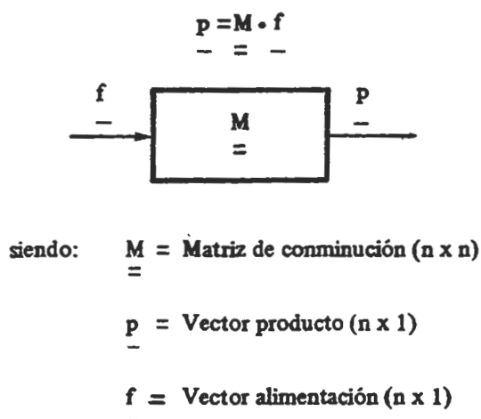
FIGURA 1.2 Representación Matemática de un Proceso de Conminución
