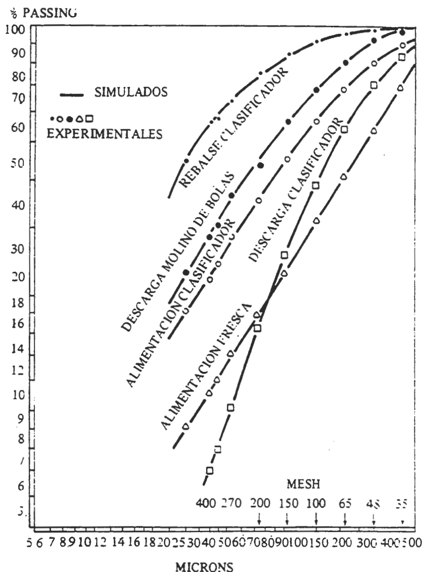
FIGURA N° 5 COMPARACION ENTRE DISTRIBUCIONES GRANULOMETRICAS SIMULADAS Y EXPERIMENTALES - PLANTA PILOTO
