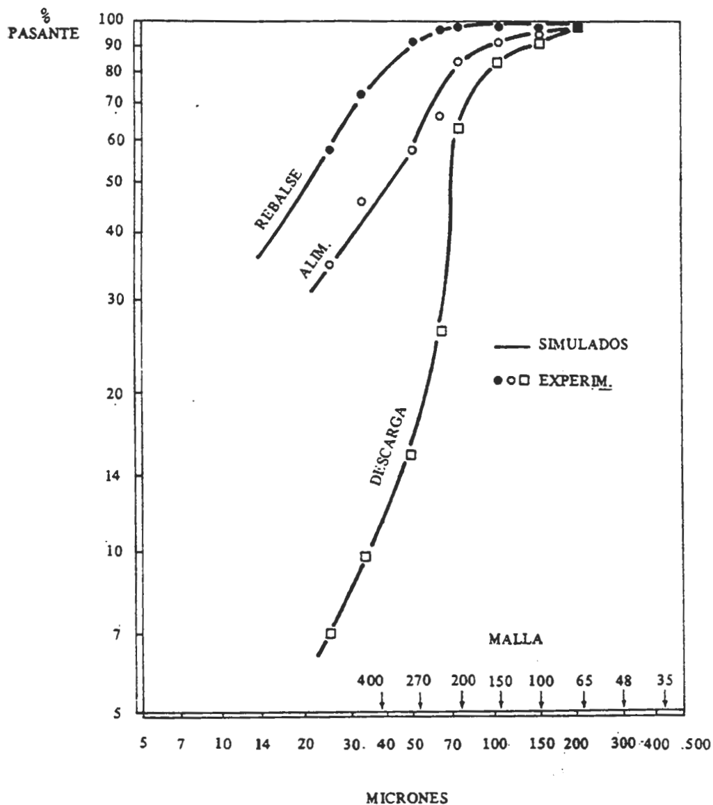
FIGURA N° 1. RESULTADOS EXPERIMENTALES Y SIMULADOS - TEST N° 1 Ciclón Krebs - 6" Diámetro Material = Arena Monazítica ( \rho_s = 3.6 ) Ensayo de Clasificación y Espesamiento - Planta Piloto.
