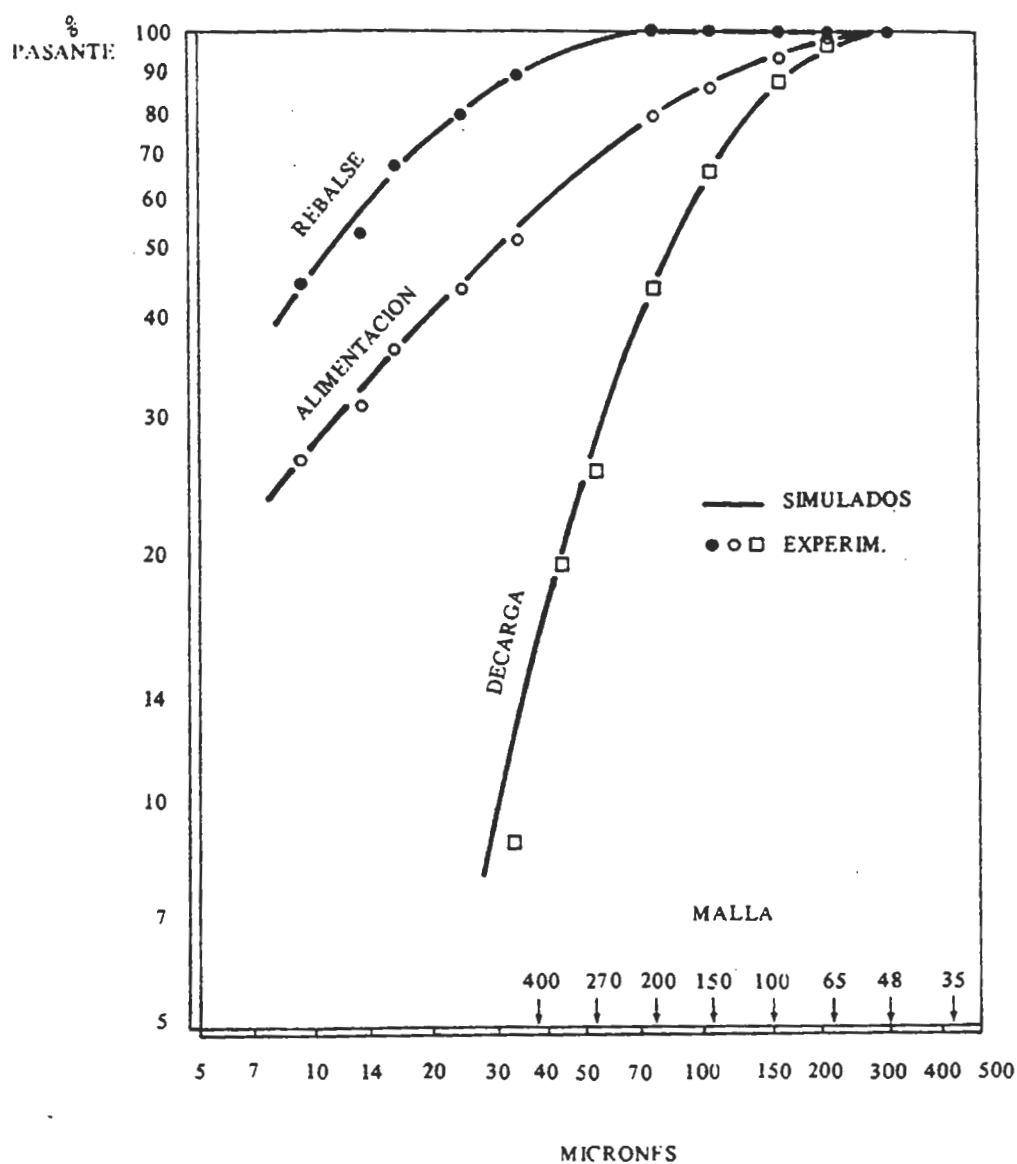
FIGURA Nº 3. RESULTADOS EXPERIMENTALES Y SIMULADOS - TEST Nº 3 Ciclón Krebs - 20" Diámetro Material = Fosfato II ( \rho_s \approx 3.2 ) Circuito Deslamado-Industrial
