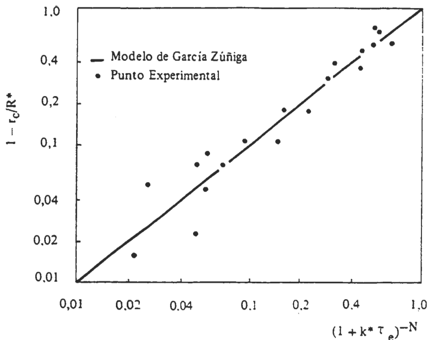
FIGURA 5.11. Gráfico Adimensional del Modelo de García Zúñiga.
