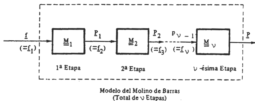
FIGURA 3.6. Representación esquemática de cada Etapa de Fractura en el Molino de Barras.
