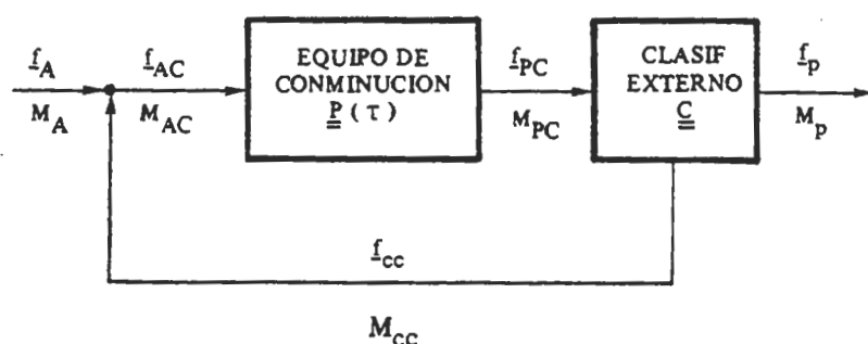
FIGURA 3.3. Representación esquemática de un circuito cerrado directo de conminución/clasificación.
