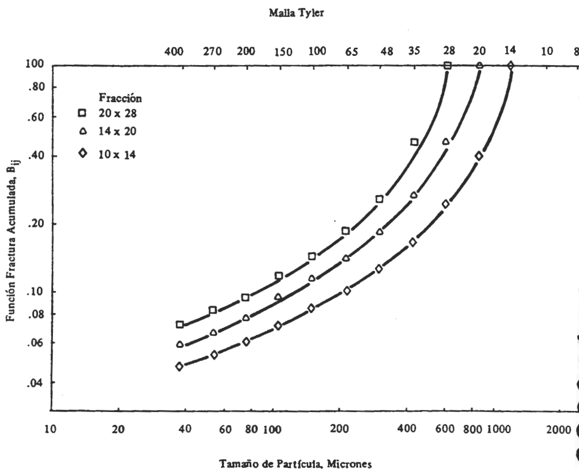
FIGURA 3.11. Función dist. de fractura acumulada versus tamaño, para 3 fracciones diferentes. Resultados extractados de la Referencia 24.
